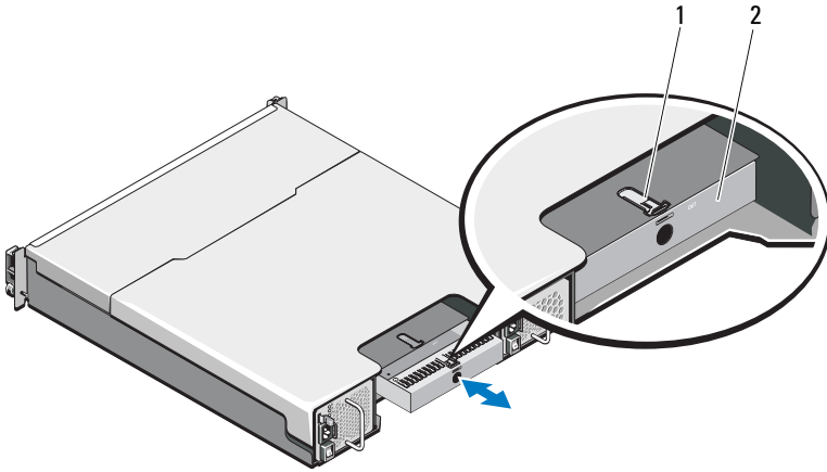
Ilustración 16-7. Extracción e instalación de un panel de relleno para el módulo de la controladora RAID
