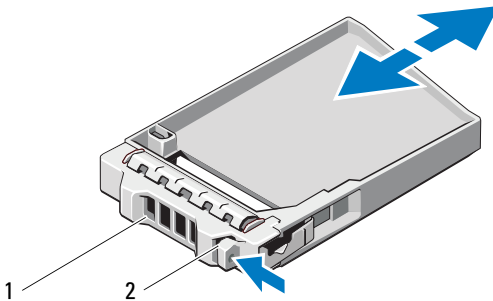
Ilustración 16-3. Extracción e instalación de una unidad de disco duro de relleno de 2,5 pulgadas (solo MD3220i).
