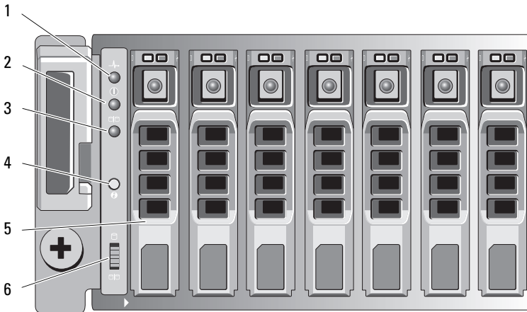
Ilustración 2-2. Indicadores y funciones del panel anterior: Dell PowerVault MD3220i
