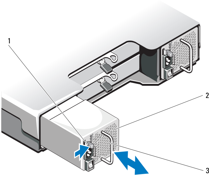
Ilustración 16-11. Extracción e instalación del módulo de suministro de energía/ventilador de enfriamiento
