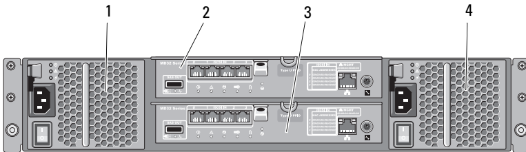
Ilustración 2-4. Indicadores y funciones del panel posterior: Dell PowerVault serie MD3200i
