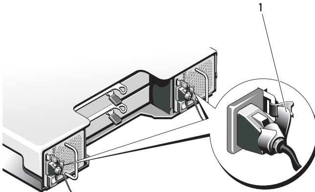
Ilustración 16-12. Fijación del cable de alimentación
