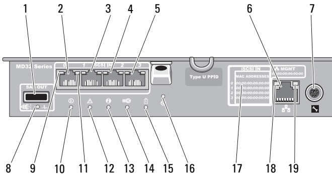
Ilustración 3-1. Módulo de la controladora RAID iSCSI serie MD3200i
