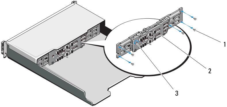
Ilustración 16-16. Extracción e instalación del plano posterior de PowerVault MD3200i
