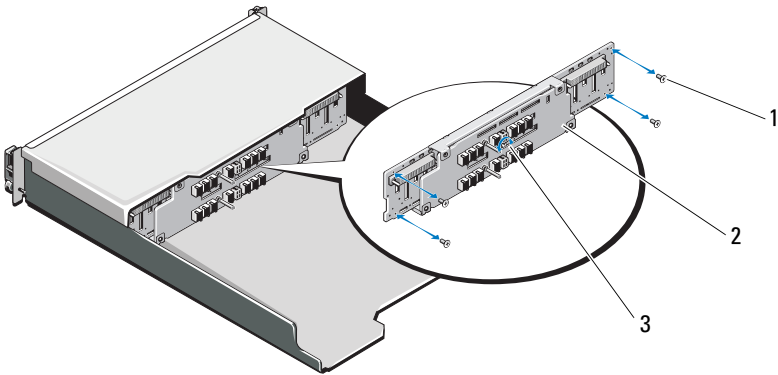
Ilustración 16-17. Extracción e instalación del plano posterior de PowerVault MD3220i
