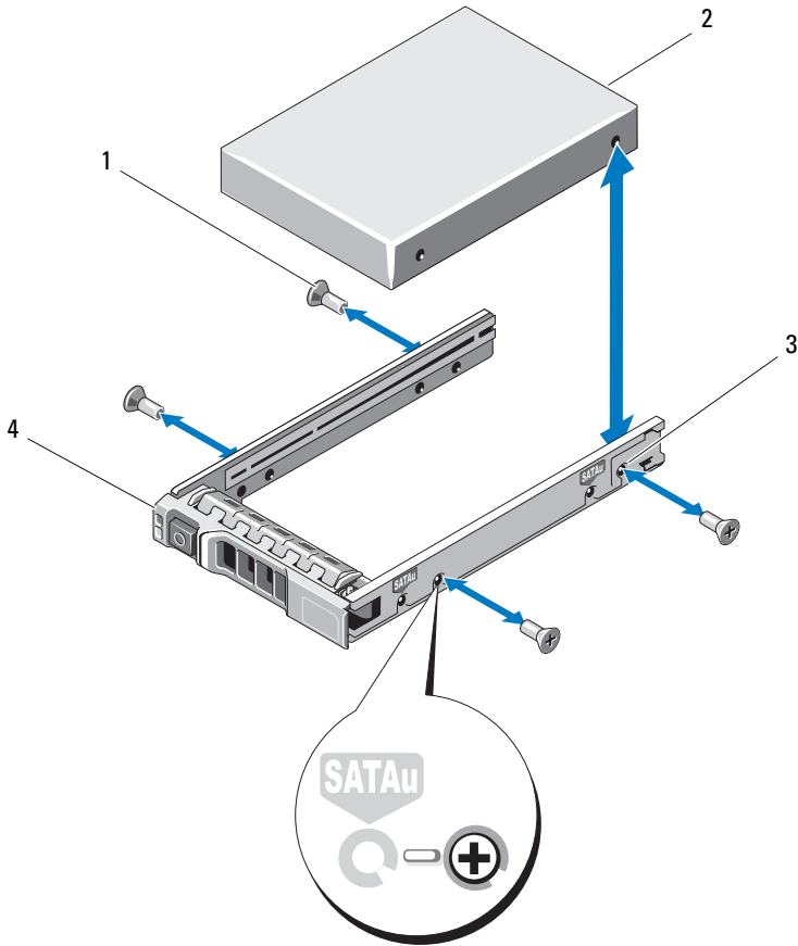
Ilustración 16-6. Extracción e instalación de una unidad de disco duro en un portaunidades de disco duro de 2,5 pulgadas
